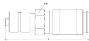
Schlauchanschluss
